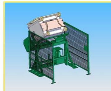
Vyklápěcí zařízení na kontejner
